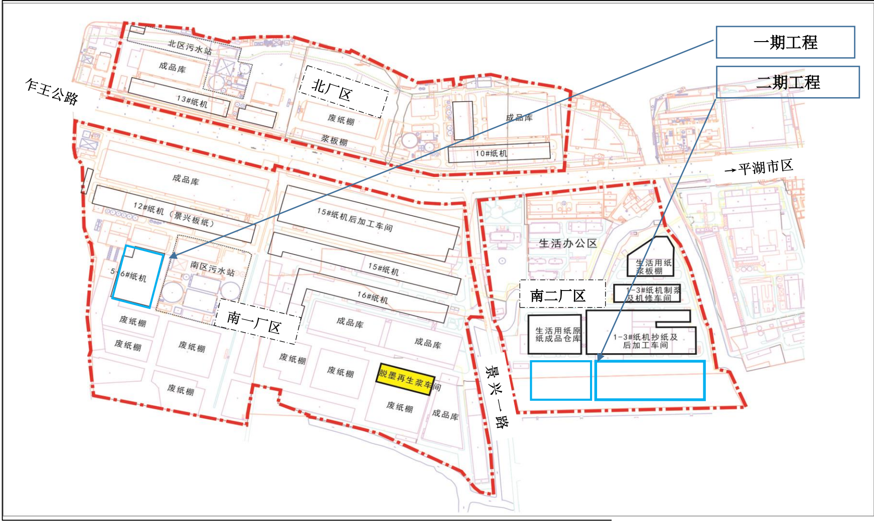
附图2 总平面布置图
